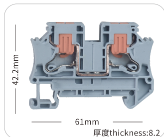
JHPTV-6
