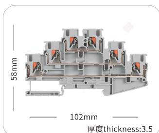
JHPT-1.5-3L
