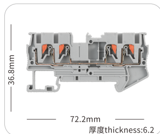
JHPT-4QT
