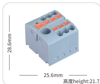
JHPTX6-6
