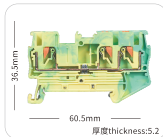
JHPT-TWPE
