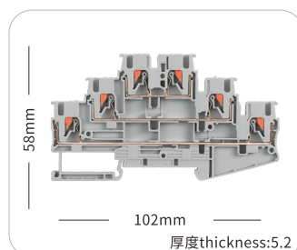
JHPT-2.5-3L
