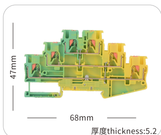
JHPT-3LPE
