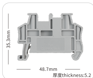
JHPT-35/5
