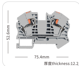
JHPT-16
