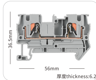
JHPT-4
