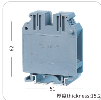
JH2UIK35
