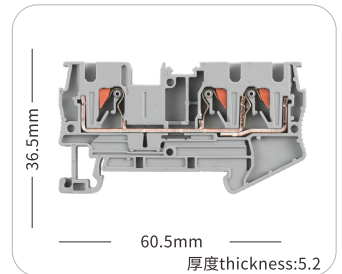
JHPT-2.5TW
