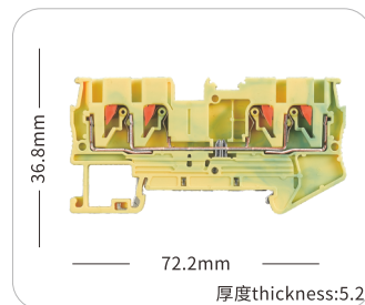
JHPT-QTPE
