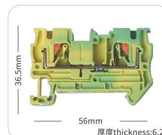
JHPT-4PE
