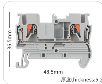
JHPT-2.5
