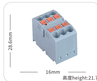
JHPTX-6
