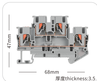
JHPT-1.5TB
