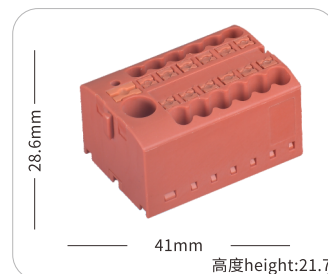
JHPTX6-12
