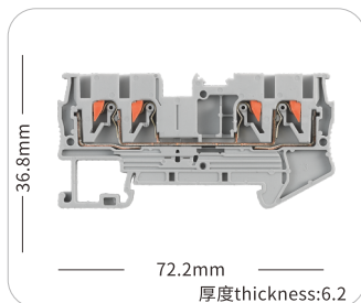
JHPT-6QT
