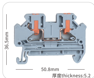
JHPTV-2.5
