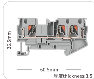
JHPT-1.5TW
