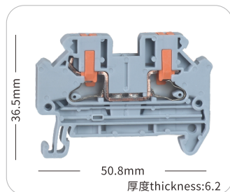
JHPTV-4
