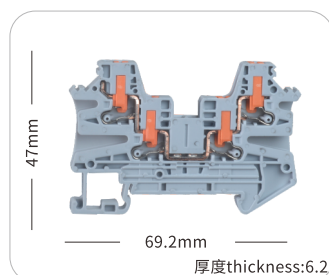
JHPTV-4QT
