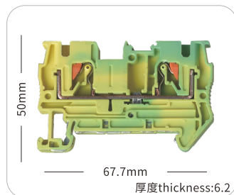
JHPT-10PE
