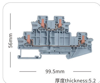
JHPTV-2.5TB
