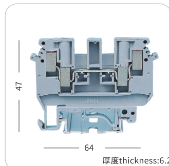
JHUDK 4
