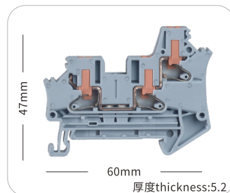
JHPTV-2.5TW
