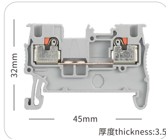
JHPT-1.5
