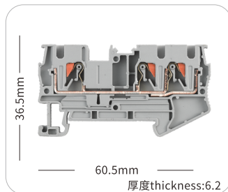
JHPT-4TW
