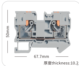
JHPT-10
