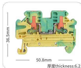
JHPTV-4PE
