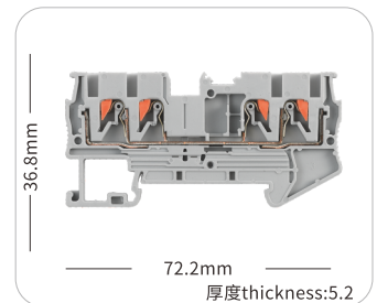
JHPT-2.5QT
