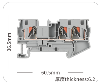
JHPT-TW
