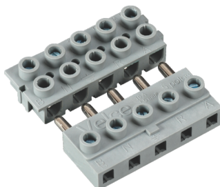
CNP-5 2.5-6mm 2
